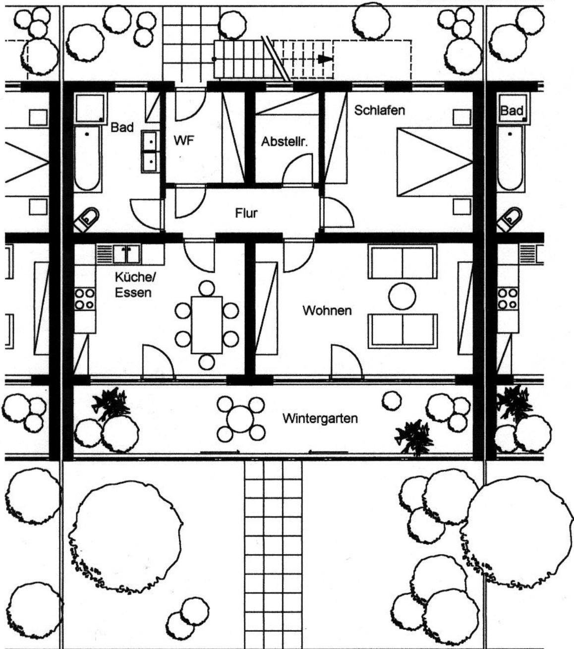
Grundriß EG M 1:100
